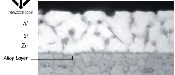
ภาพตัดขวางโครงสร้างทางจุลภาคของเหล็กเคลือบโลหะซิงคาลูม Microstructure Cross Section of ZINCALUME® steel
